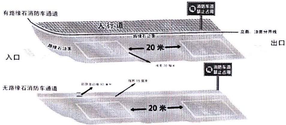
图 1：消防车通道路侧禁停标线及路面警示标志示例
