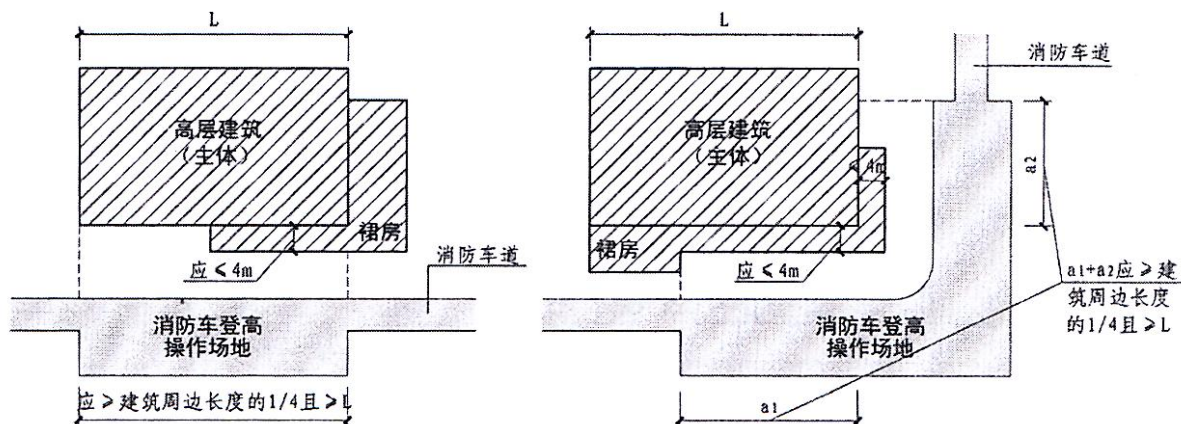
图4 消防车登高操作场地示意图
